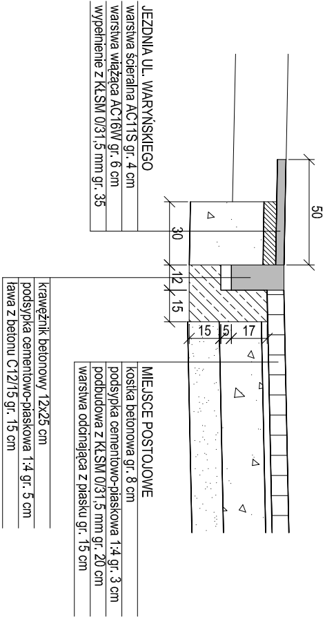
SZCZEGÓŁ KONSTRUKCYJNY "B1"
