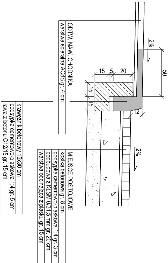
SZCZEGÓŁ KONSTRUKCYJNY "A2"
