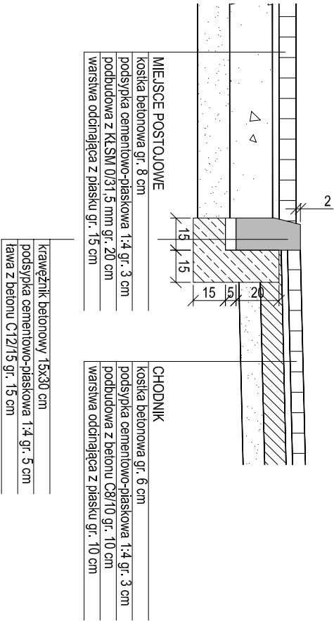
SZCZEGÓŁ KONSTRUKCYJNY "B3"
